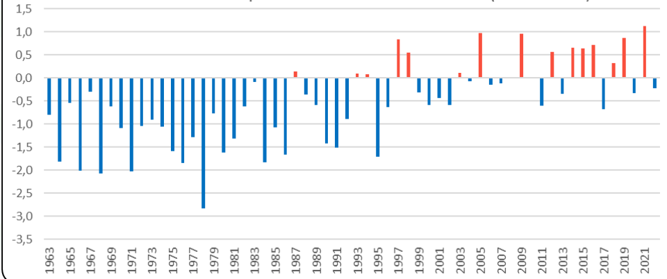
Anomalia de Temperatura Mínima - Setembro (1963-2021)
