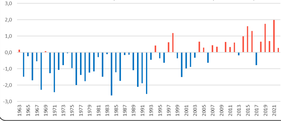
Anomalia de Temperatura Média - Setembro (1963-2021)
