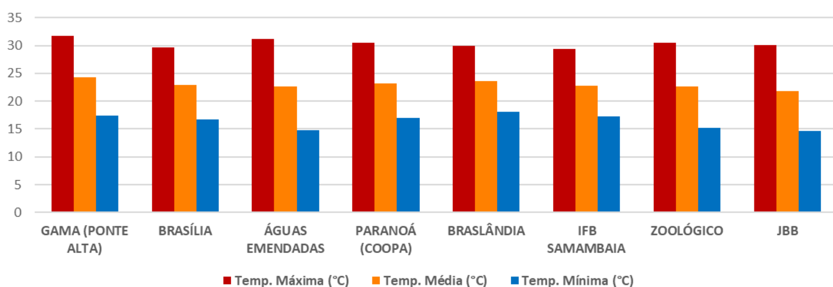
TEMPERATURAS MÉDIAS (DF) - SETEMBRO 2022
