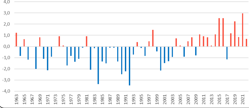
Anomalia de Temperatura Máxima - Setembro (1963-2021)
